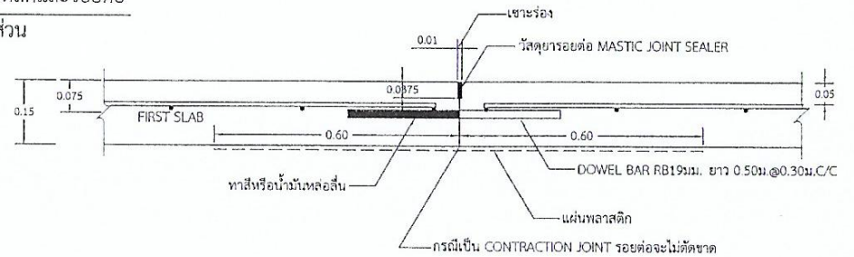
ขยายรอยต่อ CONTRACTION JOINT ไม่ระบุมาตราส่วน
